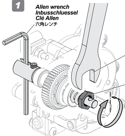
104144 Ⓐ TC Nut M7x10x3mm
